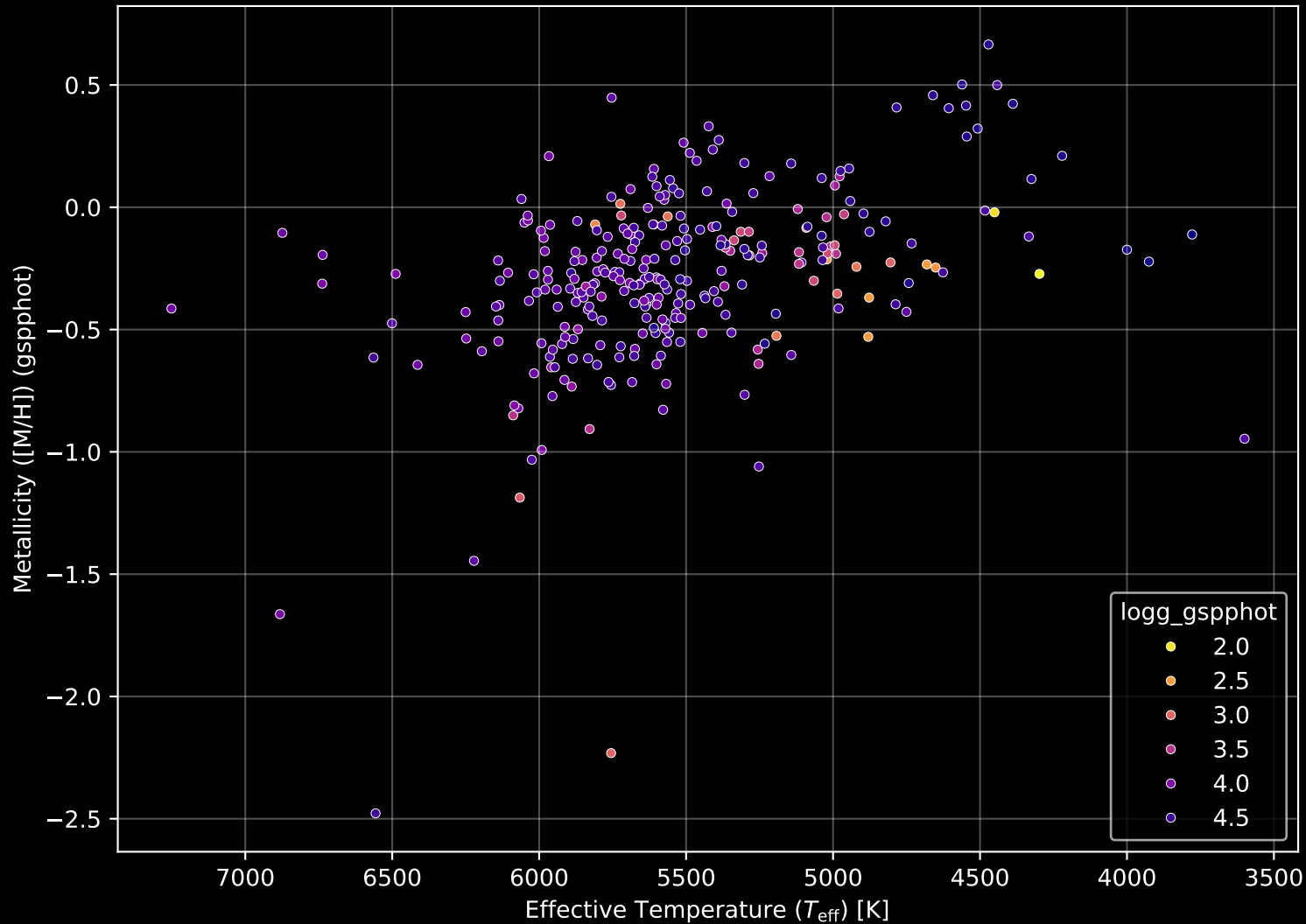
GALAH DR4 Field: [6860] Stellar Population Parameters (n= 291)
