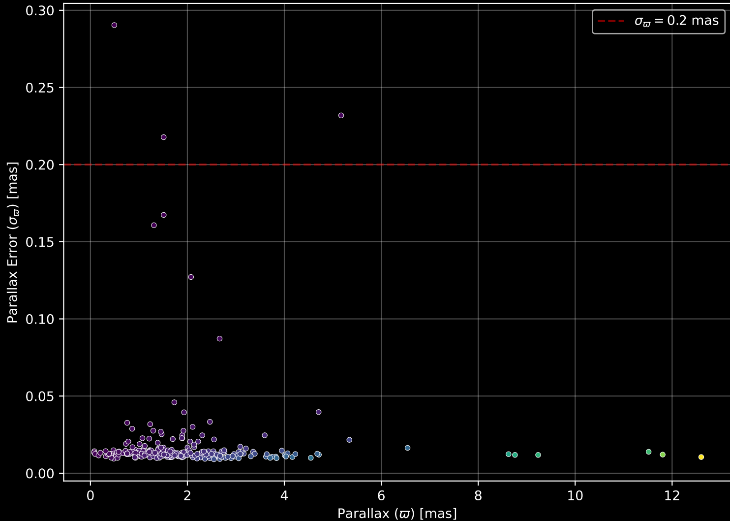
GALAH DR4 Field: [6860] Parallax Quality (n= 291)
