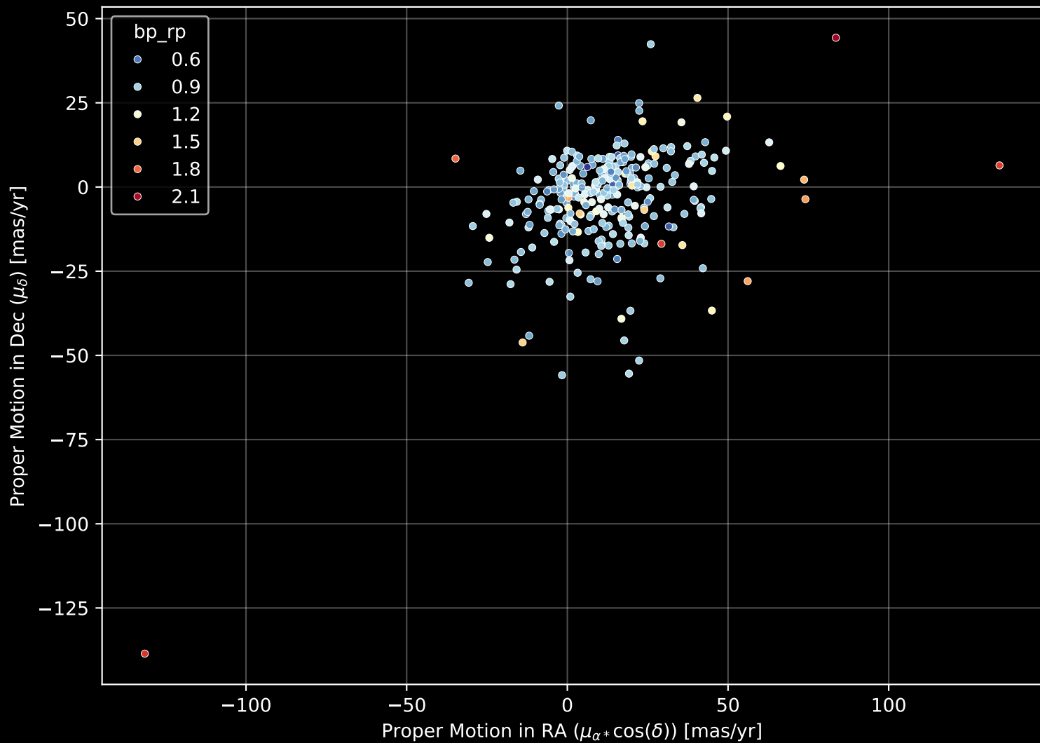
GALAH DR4 Field: [6860] Proper Motion Diagram (n= 291)
