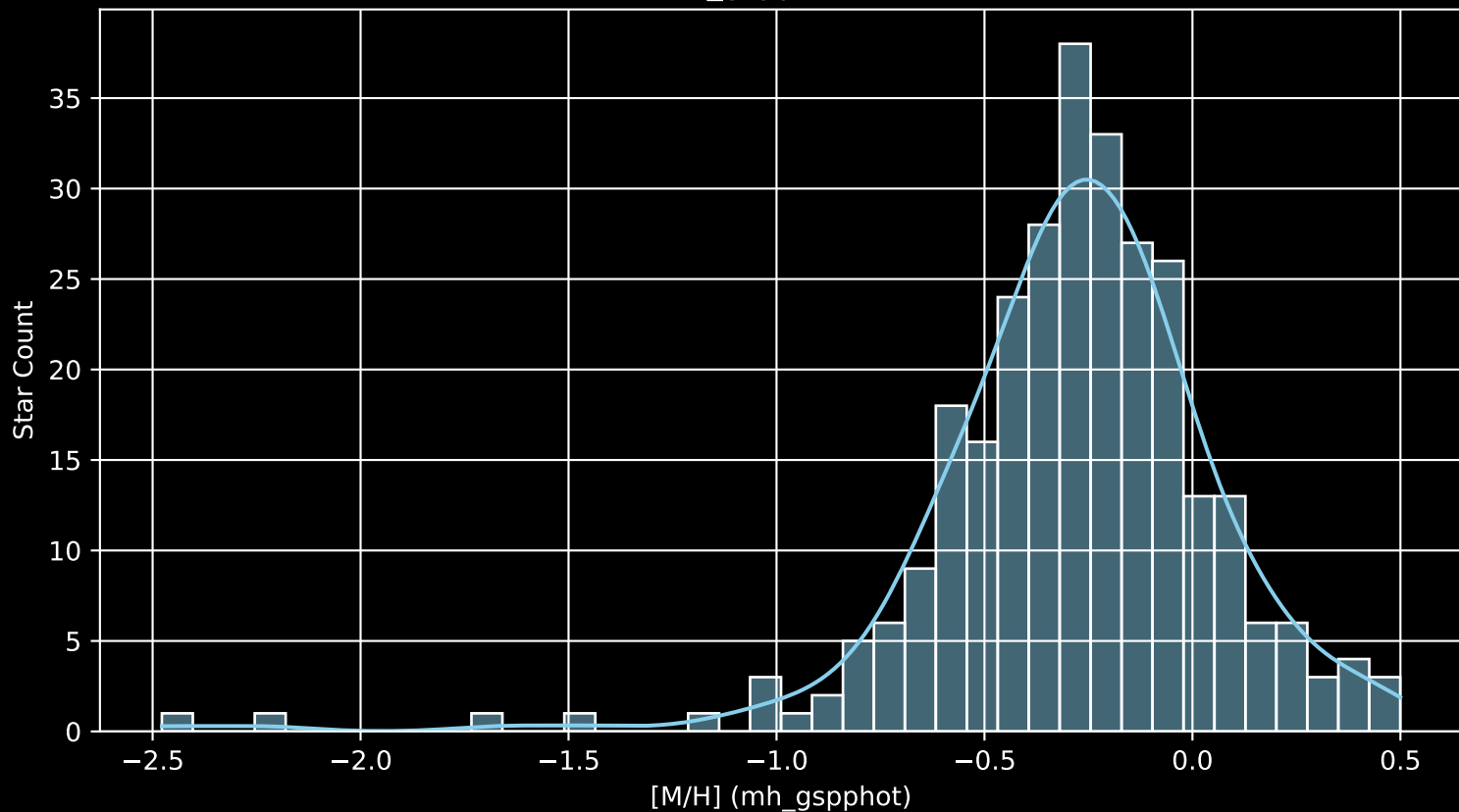
GALAH DR4 Field: [6860] [M/H] (mh_gspphot) (n= 289)
